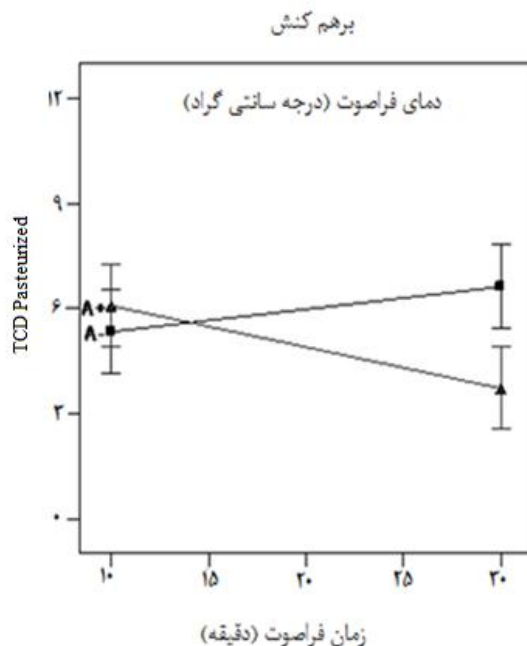
شکل ۱۱- نمودار برهم‌کنش نشان‌دهنده اثر متقابل دما و زمان روی تفاوت رنگ کل نسبت به نمونه پاستوریزه، A + نشان‌دهنده سطح بالای دما (۵۰ درجه سانتی‌گراد) و A - نشان‌دهنده سطح پایین دما (۲۵ درجه سانتی‌گراد) می‌باشد.
