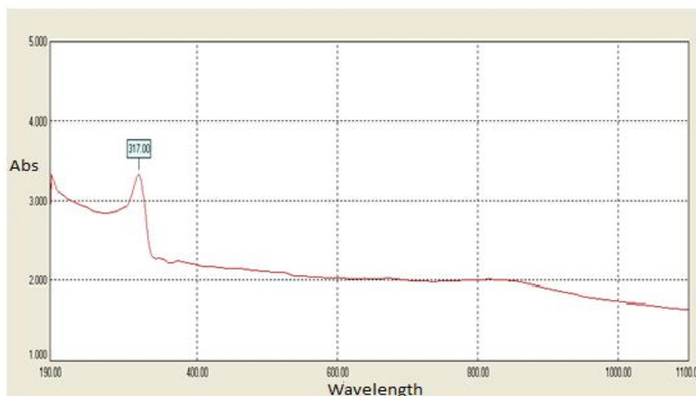
شکل ۷- طیف جذب زیرلایه متشکل از نانو سیم‌های نقره در محدوده ۱۱۰۰-۱۹۰ نانومتر
