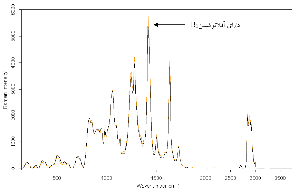
شکل ۴- میانگین طیف‌های رامان حاصل از نمونه‌های خمیری پسته عاری و حاوی آفلاتوکسین B 1 با غلظت ۵ میکروگرم در لیتر
