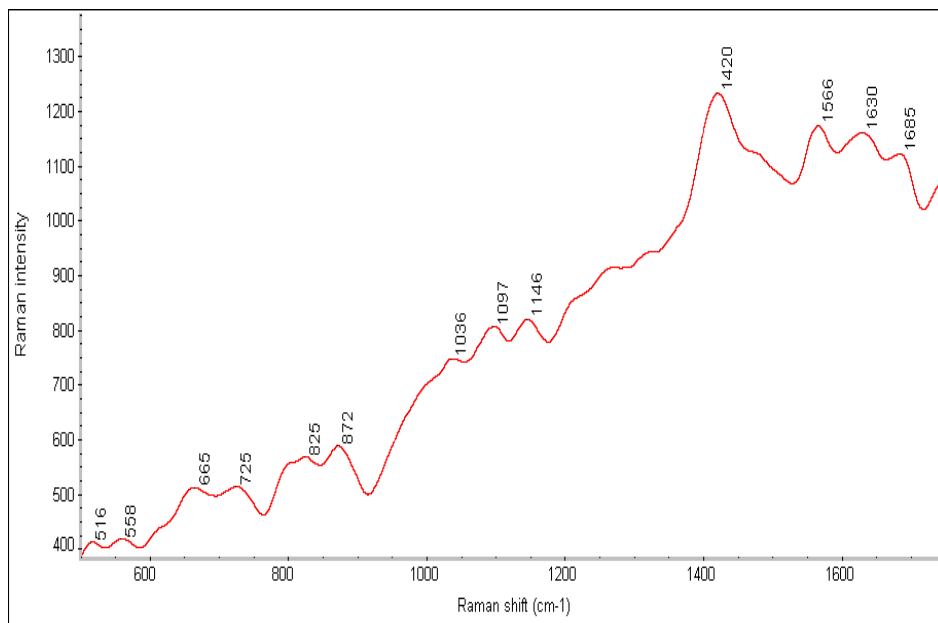
شکل ۱۰- طیف آفلاتوکسین B 1 (غلظت ۵ میکروگرم در لیتر) با استفاده از زیرلایه متشکل از کلئید نانوذرات نقره روی شیشه
