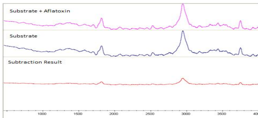
شکل ۶- تفاضل میانگین طیف‌های زمینه (زیرلایه) از میانگین طیف‌های زیرلایه‌های حاوی آفلاتوکسین B 1 (۵ میکروگرم در لیتر)
