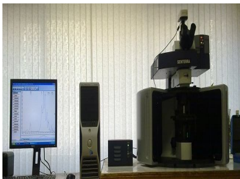
شکل ۲- سامانه طیف سنجی سنترابروکر
