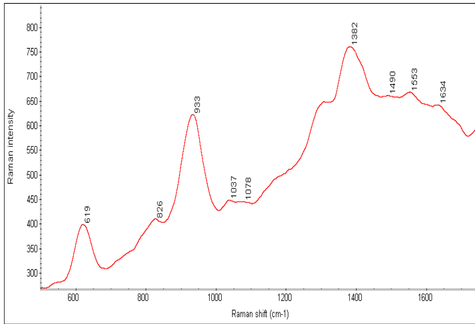
شکل ۹- طیف آفلاتوکسین B 1 (غلظت ۱۰۰ میکروگرم در لیتر) با استفاده از زیرلایه متشکل از کلئید نانوذرات نقره روی شیشه
