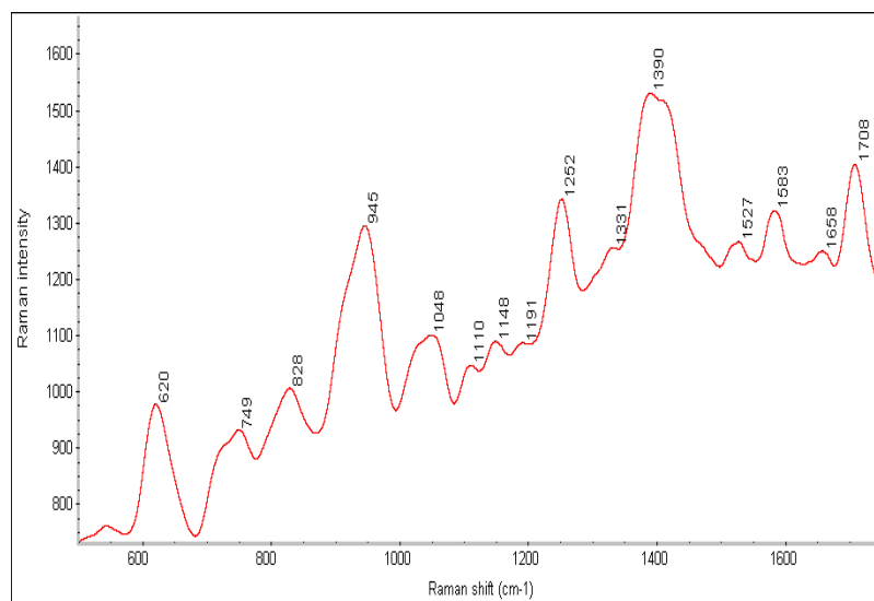
شکل ۸- طیف آفلاتوکسین B 1 (غلظت ۱۰۰۰ میکروگرم در لیتر) بدست آمده با استفاده از زیرلایه متشکل از کلئید نانوذرات نقره روی شیشه
