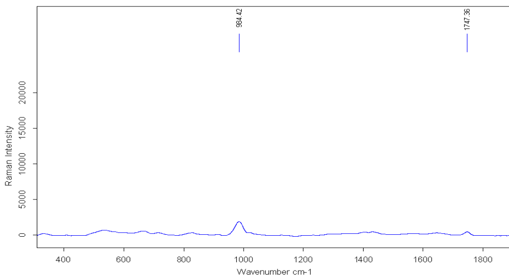
شکل ۵- طیف حاصل از تفاضل میانگین طیف‌های زمینه (زیرلایه) از میانگین طیف‌های زیرلایه + آفلاتوکسین B 1 (۵ میکروگرم در لیتر)
