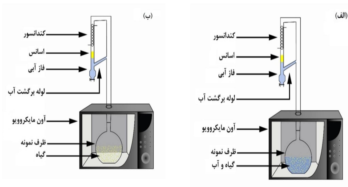
شکل ۱- دستگاه استخراج اسانس با روش‌های (الف) تقطیر با آب به کمک میکروویو و (ب) میکروویو بدون حلال.
