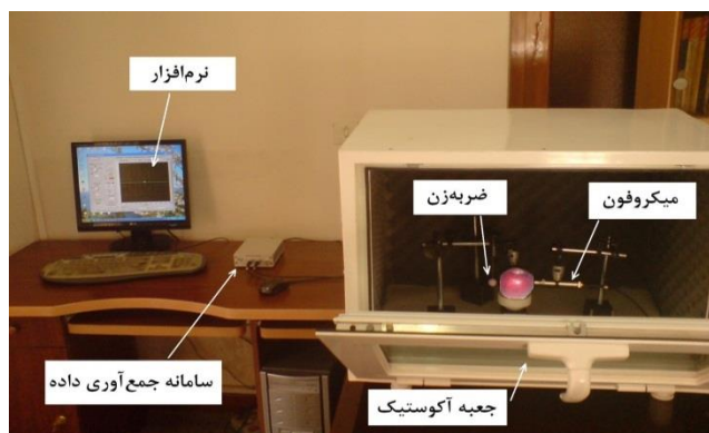
شکل ۱ - جعبه آکوستیک
