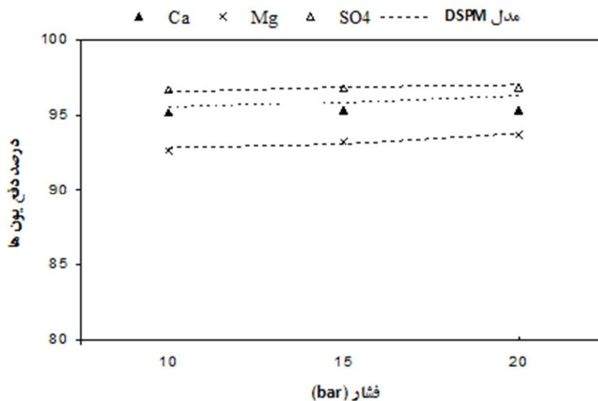
شکل 8- درصد دفع یون‌های دو ظرفیتی در طی نانوفیلتراسیون آب پرس تفاله چغندر قند در اختلاف فشارهای عرضی مختلف (نمادها، داده های تجربی و خط چین، نتایج مدلسازی فیزیکی)
