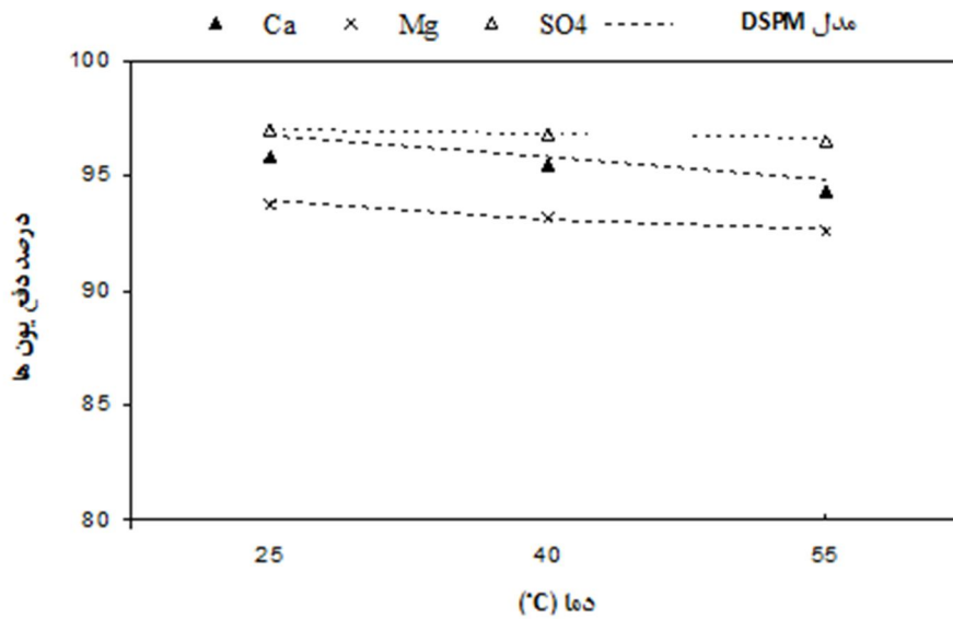
شکل 6- درصد دفع یونهای دو ظرفیتی در طی نانوفیلتراسیون آب پرس تفاله چغندر قند در دماهای مختلف (نمادها، داده‌های تجربی و خط چین، نتایج مدلسازی فیزیکی)
