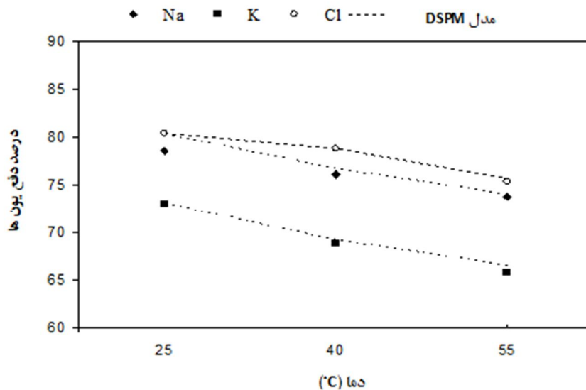
شکل 5- درصد دفع یون های تک ظرفیتی در طی نانوفیلتراسیون آب پرس تفاله چغندر قند در دماهای مختلف (نمادها، داده های تجربی و خط چین، نتایج مدلسازی فیزیکی)
