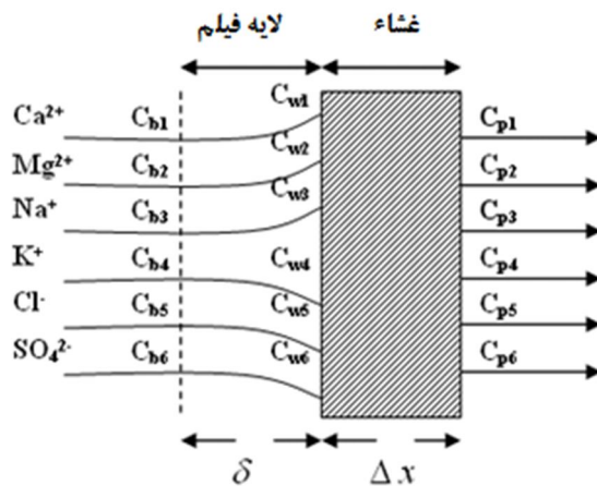
شکل 1 - عملکرد غشاء در دفع یون ها در طی نانوفیلتراسیون آب پرس تفاله
