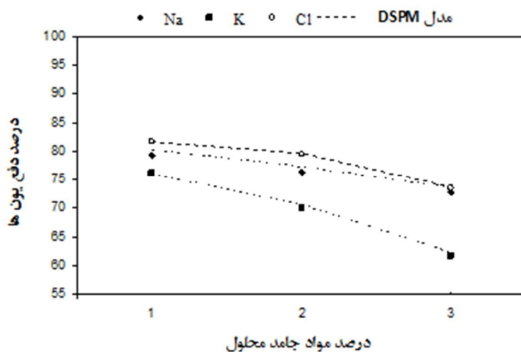
شکل 3- درصد دفع یون های تک ظرفیتی در طی نانوفیلتراسیون آب پرس تفاله چغندر قند در غلظت های مختلف (نمادها، داده های تجربی و خط چین، نتایج مدلسازی فیزیکی)
