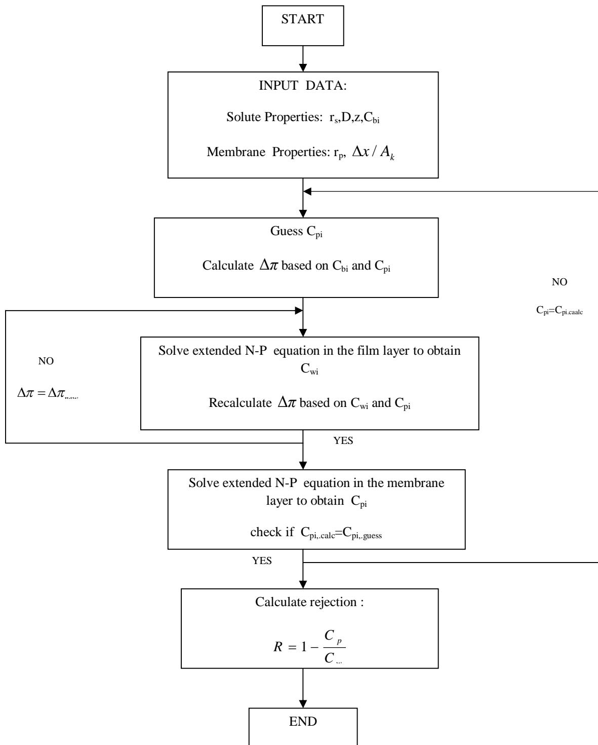
شکل 2- دیاگرام الگوریتم مدل‌سازی DSPM آب پرس تفاله چغندر قند
