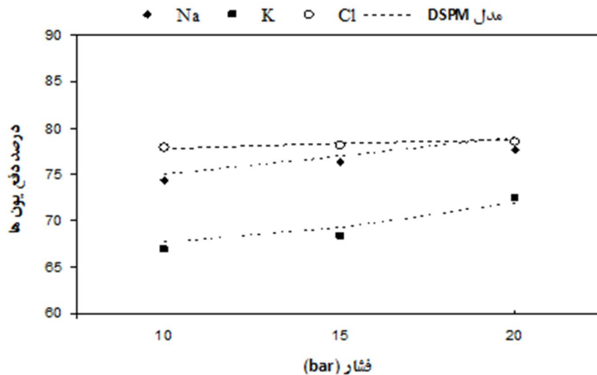
شکل 7- درصد دفع یون‌های تک ظرفیتی در طی نانوفیلتراسیون آب پرس تفاله چغندر قند در اختلاف فشارهای عرضی مختلف (نمادها، داده های تجربی و خط چین، نتایج مدلسازی فیزیکی)
