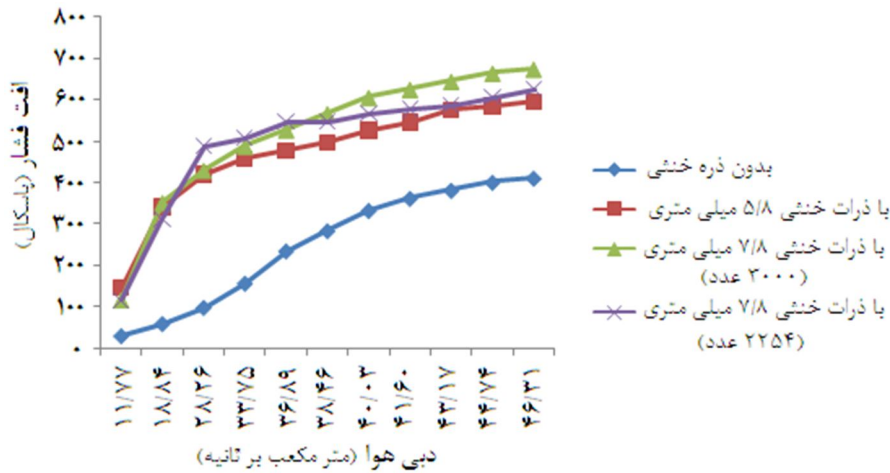
شکل 2- تغییرات افت فشار بین قسمت ورودی و خروجی بستر در 4 حالت (اعداد مربوط به دبی هوا در 10^3 ضرب شده اند)
