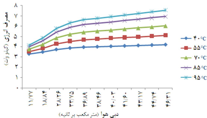
شکل 4- مصرف انرژی (در هر ساعت) در دبی‌های حجمی و دماهای مختلف (اعداد مربوط به دبی هوا در 10^3 ضرب شده اند)
