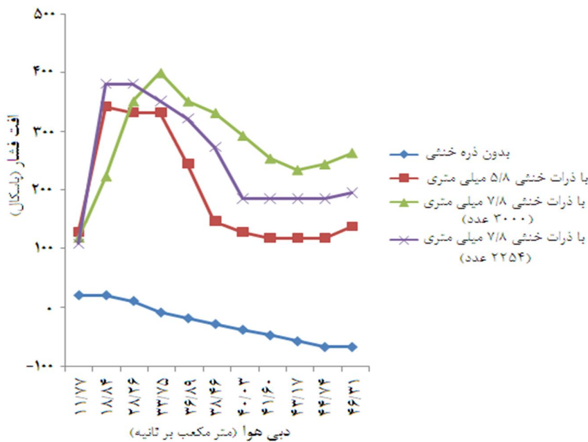
شکل 3- تغییرات افت فشار بین قسمت ورودی و میانی بستر در 4 حالت (اعداد مربوط به دبی هوا در 10^3 ضرب شده‌اند)
