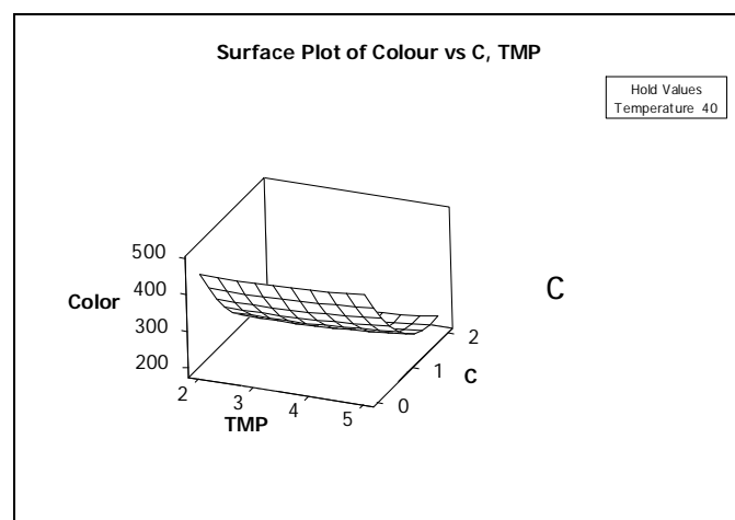
شکل 4- تاثیر دما، فشار و غلظت عامل فعال سطحی بر میزان رنگ جریان تراوه
