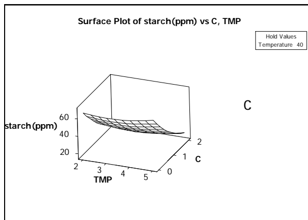
شکل 6- تاثیر دما، فشار و غلظت عامل فعال سطحی بر میزان نشاسته جریان تراوه
