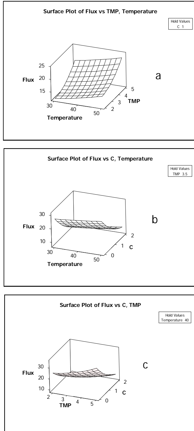
شکل 2- تأثیر دما، فشار و غلظت عامل فعال سطحی بر میزان شار جریان تراوه
