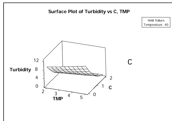
شکل 3- تاثیر دما، فشار و غلظت عامل فعال سطحی بر میزان کدورت جریان تراوه
