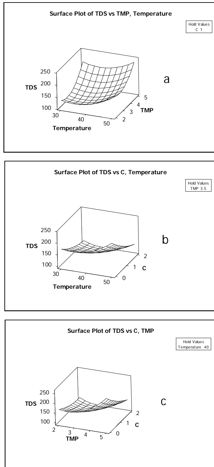
شکل 5- تاثیر دما، فشار و غلظت عامل فعال سطحی بر TDS جریان تراوه
