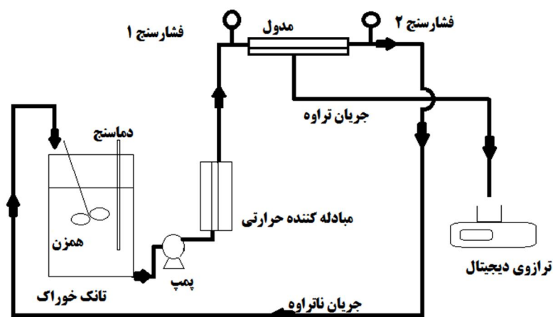
شکل 1- شماتیک پایلوت غشایی فرابالایش برای تصفیه شکر خام به روش MEUF
