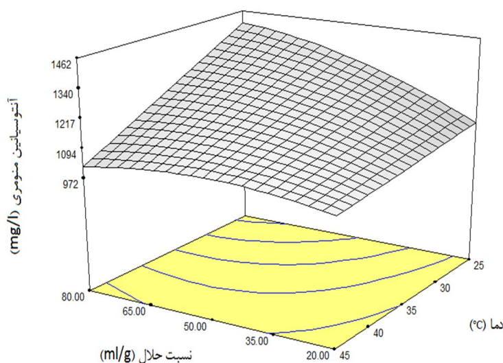
شکل 3- نمودار سطح پاسخ میزان آنتوسیانین در مقابل دو متغیر دما - نسبت حلال پس از زمان 16 ساعت و 50 درصد اتانول
