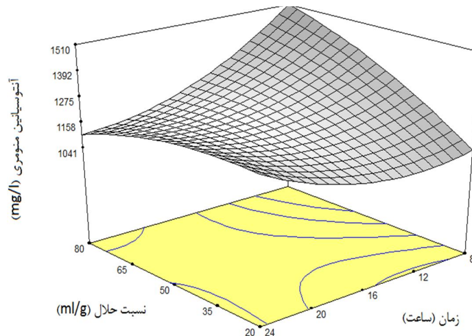
شکل 5- نمودار سطح پاسخ میزان آنتوسیانین در مقابل دو متغیر زمان - نسبت حلال در دمای 35 درجه سانتی‌گراد و درصد اتانول 50 درصد
