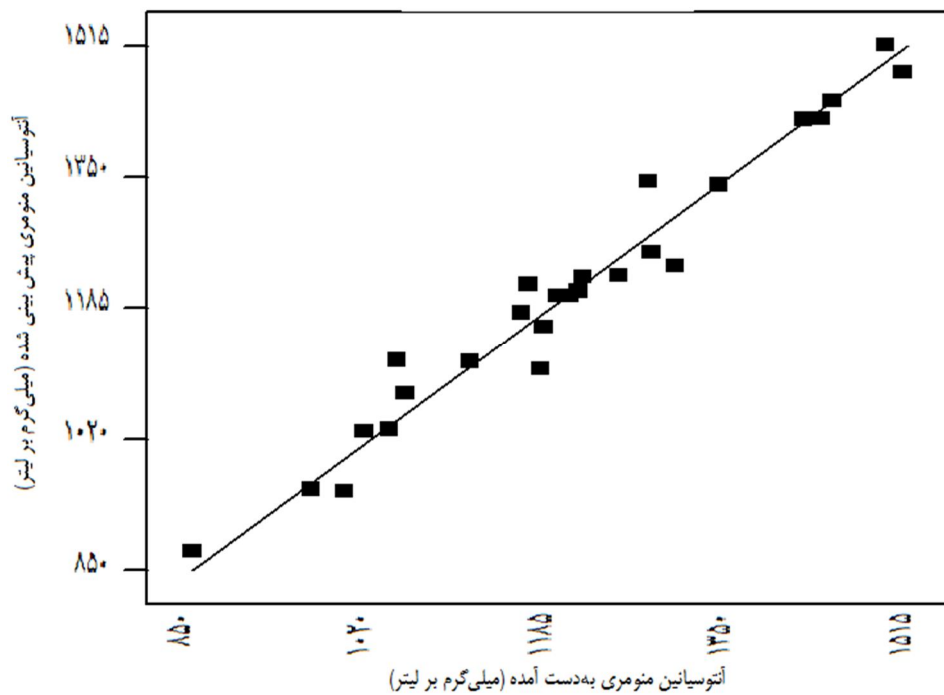
شکل 1- مقایسه میزان آنتوسیانین پیش بینی شده در مدل و مقادیر واقعی به دست آمده در روش استخراج سنتی با حلال
