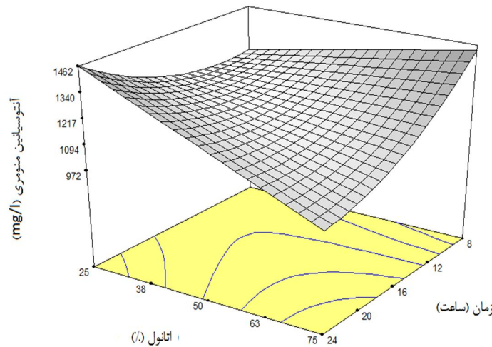
شکل 6- نمودار سطح پاسخ میزان آنتوسیانین در مقابل دو متغیر زمان-درصد اتانول در دمای 35 درجه سانتی‌گراد و نسبت حلال 55 میلی‌لیتر بر گرم نمونه
