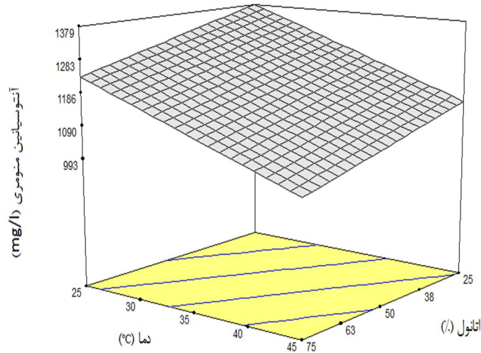
شکل 4- نمودار سطح پاسخ میزان آنتوسیانین در مقابل دو متغیر درصد اتانول - دما در زمان 16 ساعت و نسبت حلال 50 میلی‌لیتر بر گرم نمونه
