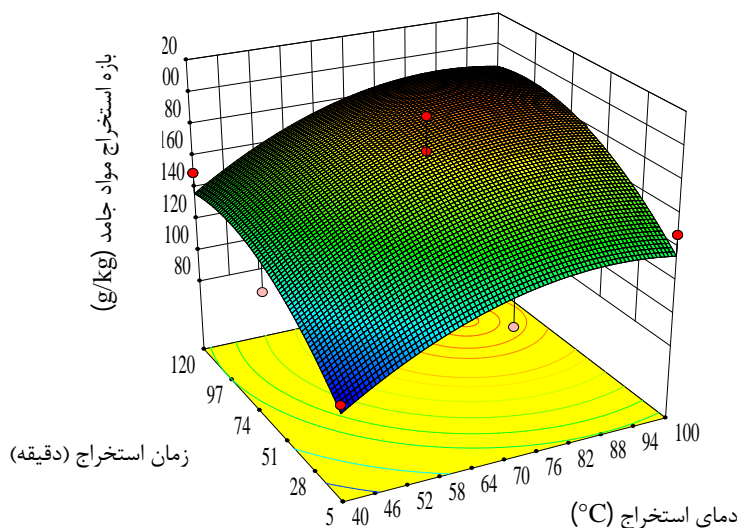
شکل 1- نمودار سه بعدی، اثر همزمان دما و زمان استخراج را بر بازده استخراج مواد جامد چای سبز
