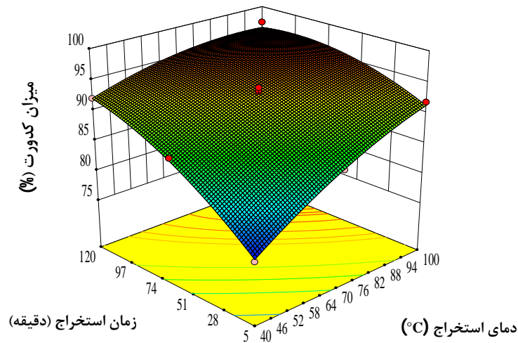
شکل 3- نمودار سه بعدی، اثر همزمان دما و زمان استخراج بر میزان کدورت چای سبز
