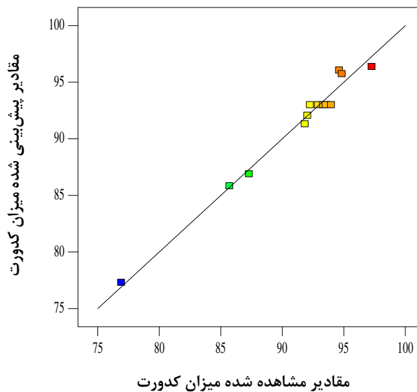
شکل 4- مقایسه مقادیر مشاهده شده و پیش‌بینی شده میزان کدورت چای سبز
