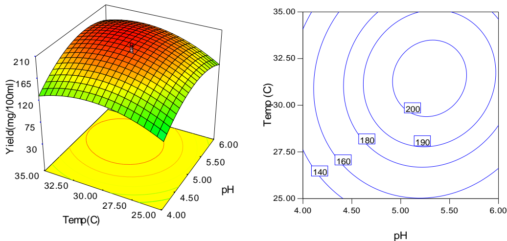
شکل 3- منحنی‌های سطح پاسخ تراز و سه بعدی اثر تداخلی دما و pH بر میزان راندمان مانان
