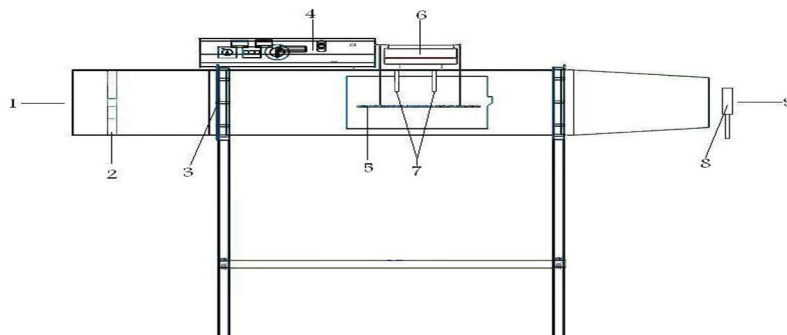
شکل 1- شماتیک خشک کن مورد استفاده: (1) ورودی هوا؛ (2) فن؛ (3) گرمکن؛ (4) تابلو فرمان یا محفظه کنترل کننده دما و سرعت؛ (5) سینی سوراخ دار؛ (6) ترازوی دیجیتال؛ (7) سنسور رطوبت؛ (8) سرعت سنج دیجیتالی هوا؛ (9) خروجی هوا
