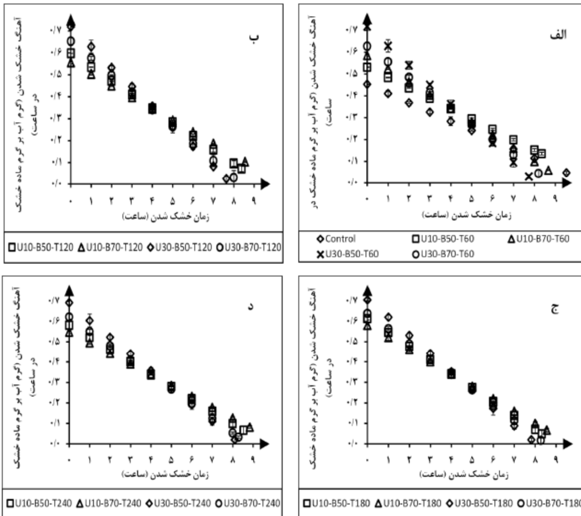
شکل 3- (الف-د) - آهنگ خشک‌شدن تیمارهای مختلف بر اساس جدول 1 طی خشک‌شدن
