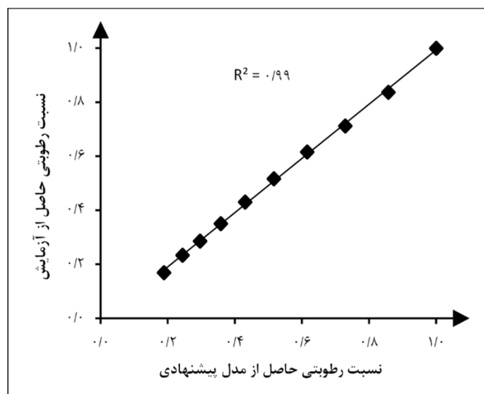
شکل 5- برازش داده‌های نسبت رطوبت حاصل از آزمایش با داده‌های حاصل از مدل پیشنهادی (مدل 6)
