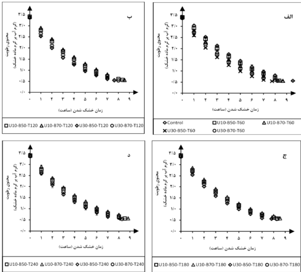
شکل 2- (الف-د) - محتوی رطوبت طی خشک‌شدن تیمارهای مختلف بر اساس جدول 1
