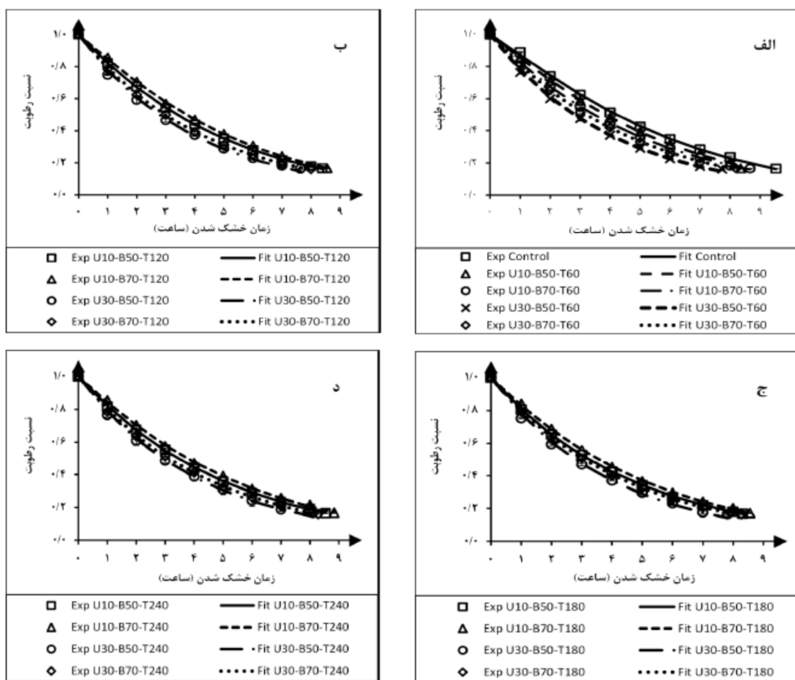
شکل 4 (الف-د) - نسبت رطوبت طی خشک‌شدن تیمارهای مختلف بر اساس جدول 1 و برازش آن‌ها با مدل پیشنهادی (مدل 6). در این شکل، Exp، داده‌های حاصل از آزمایش و Fit، داده‌های حاصل از برازش را نشان می‌دهد.
