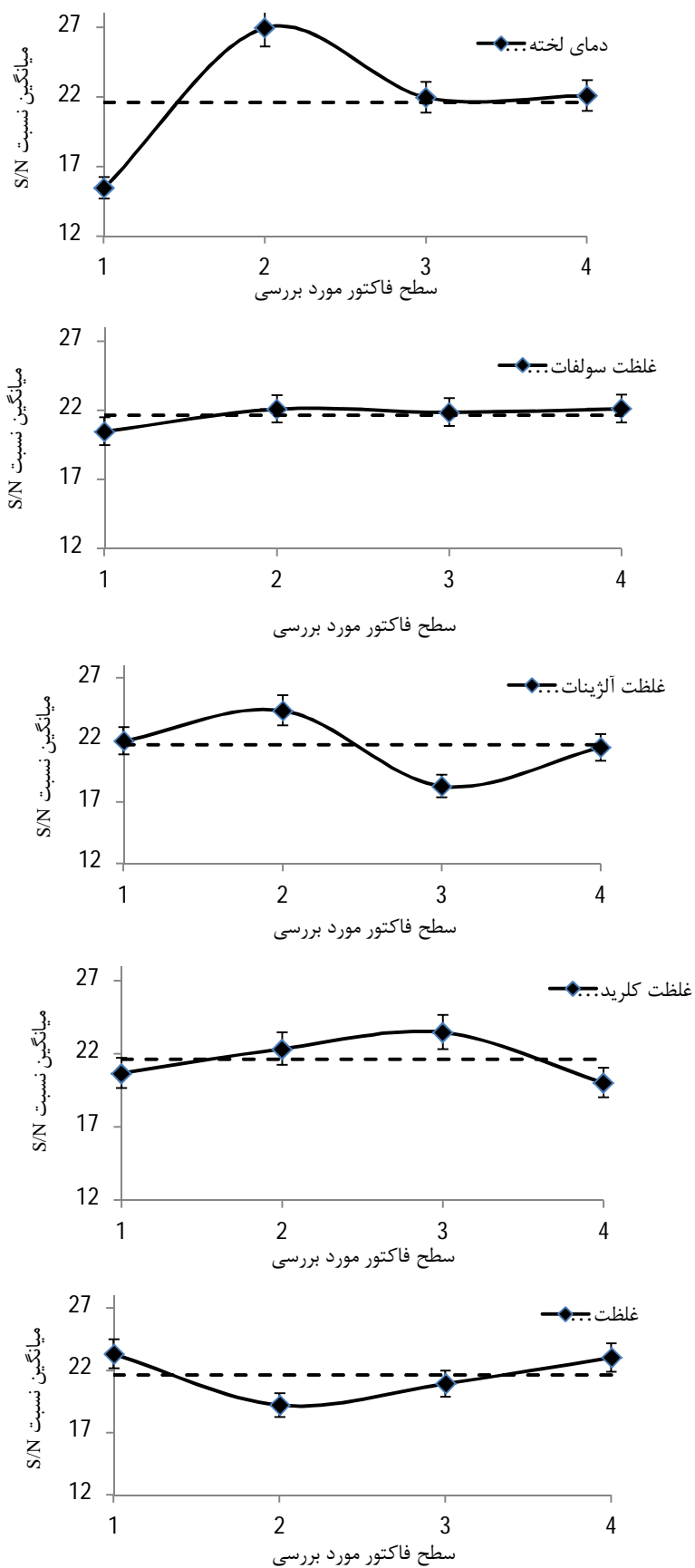
شکل 1- نمودارهای میانگین نسبت S/N سطوح مختلف هر یک از فاکتورهای موثر بر کاهش میزان اکسیژن مورد نیاز بیولوژیکی
