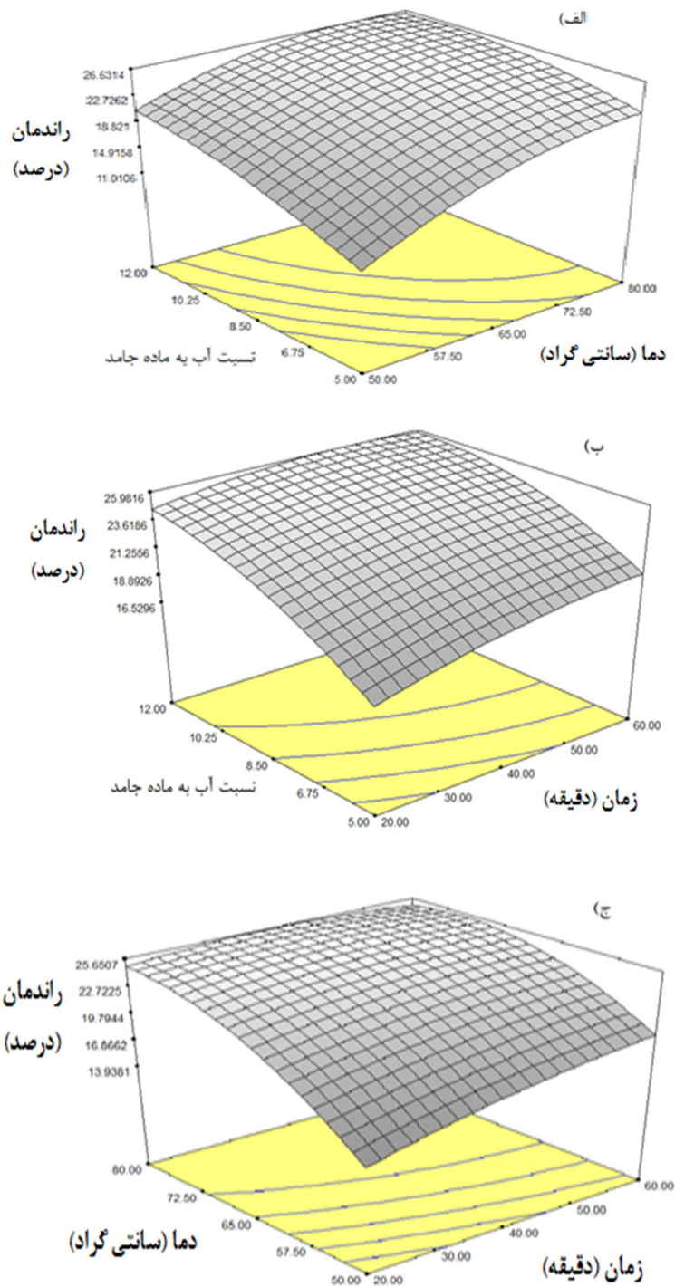
شکل 1- نمایش نمودار سه‌بعدی اثر هم‌زمان دو متغیر نسبت آب به ماده جامد و دما (الف)، نسبت آب به ماده جامد و زمان (ب)، دما و زمان (ج) بر راندمان استخراج.
