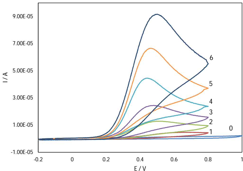
شکل 2- ولتاموگرام نمونه‌های استاندارد اسکوربیک اسید
