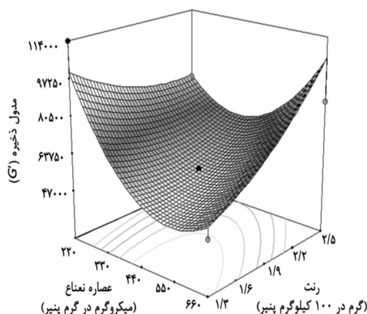
شکل ۲- تغییرات میزان مدول ذخیره در مقادیر مختلف عصاره نعناع و آنزیم رنت در نمونه‌های حاوی ۲ گرم استارتر (در ۱۰۰ گرم رنتیت) نگهداری شده تا ۳۰ روز
